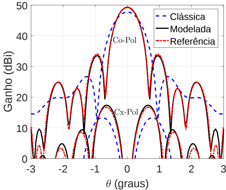
Figura 2.17 – Diagramas de radiação no plano diagonal \phi = 45^\circ das configurações ADC clássica (linhas tracejadas) e sintetizada (linhas sólidas) para o estudo de caso A.1, juntamente com o diagrama de radiação da antenna modelada de (Moreira; Bergmann, 2011).
