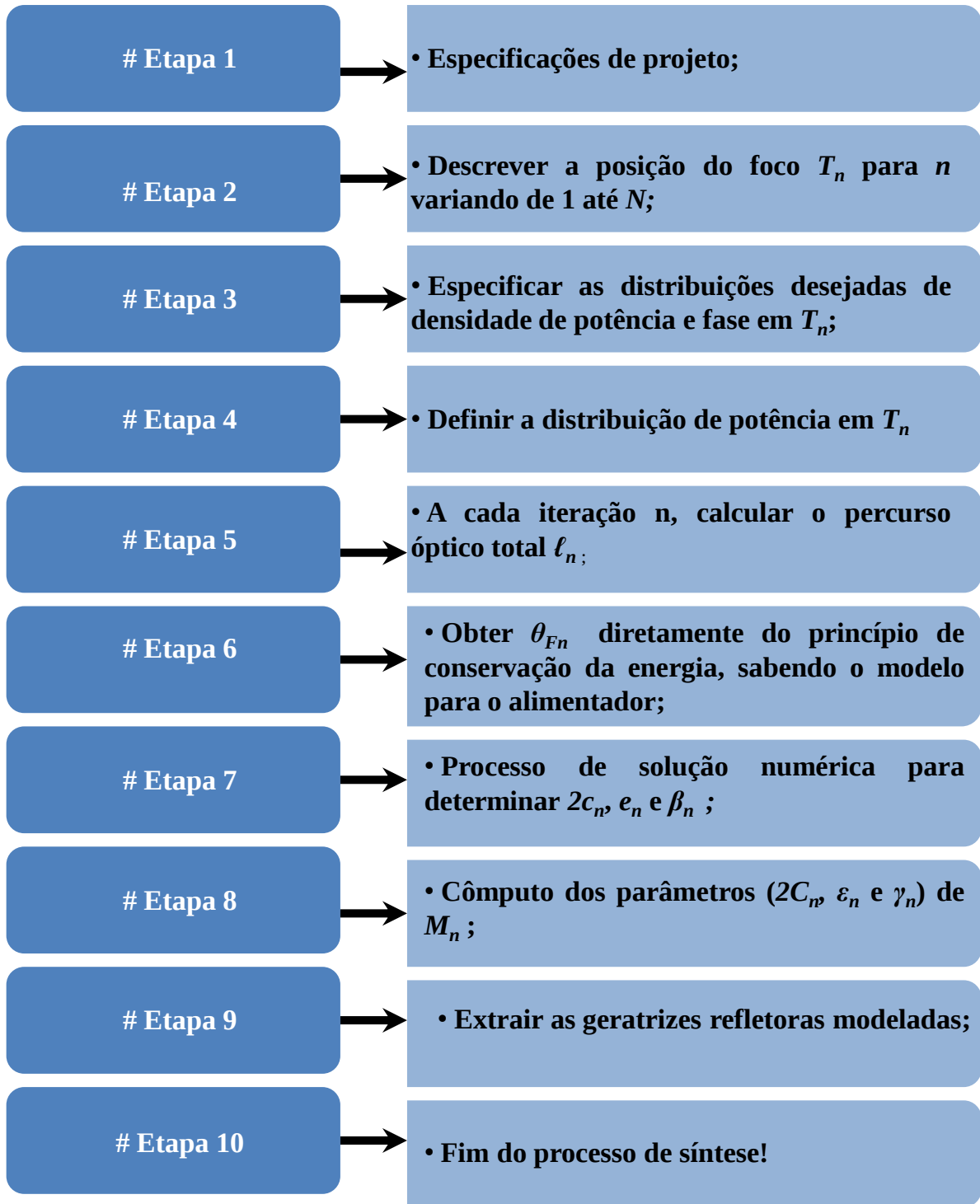
Figura 2.13 – Etapas do procedimento de síntese das configurações duplo-refleloras circularmente simétricas de eixo deslocado.
