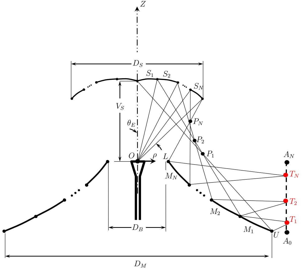
Figura 4.9 – Antena duplo-refletores para cobertura omnidirecional baseada em uma configuração OADE, com as geratrizes refletoras modeladas pela concatenação contínua de seções cônicas, sendo a geratriz do refletor principal representada por elipses.
