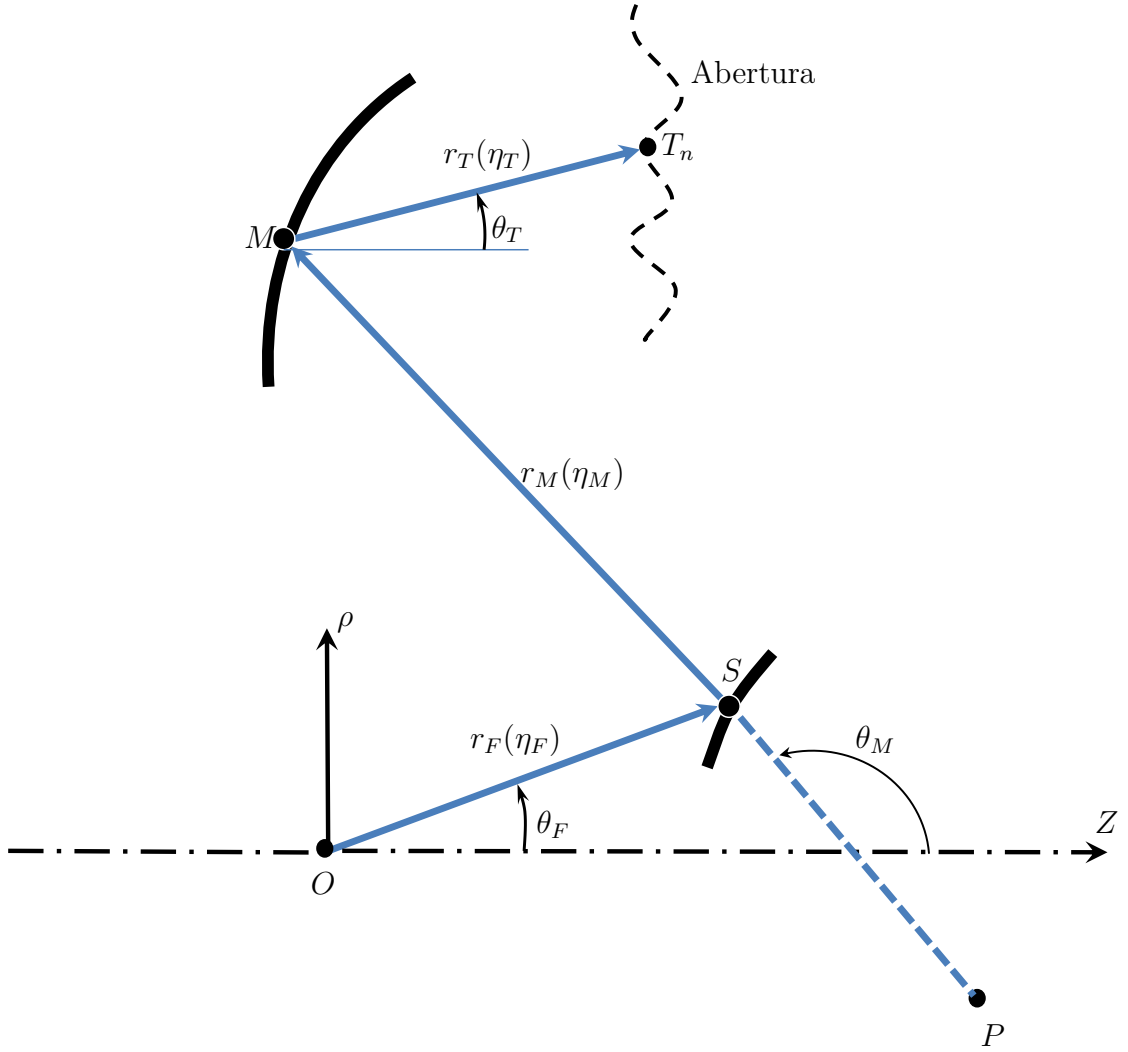
Figura 2.9 – Percurso óptico total do raio desde o centro de fase do alimentador (origem O ) até o foco T_n na abertura em uma configuração duplo-refletora simétrica de eixo deslocado.
