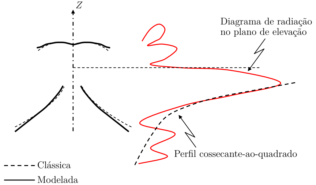
Figura 5.1 – Exemplo de um diagrama de radiação com perfil cossecante-ao-quadrado no plano de elevação gerado por uma configuração duplo-refletora omnidirecional modelada.
