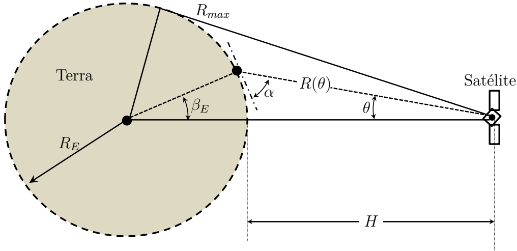
Figura 3.3 – Esquema geométrico do satélite em relação a Terra ilustrando as características de um diagrama de radiação isoflux (sem escala).
