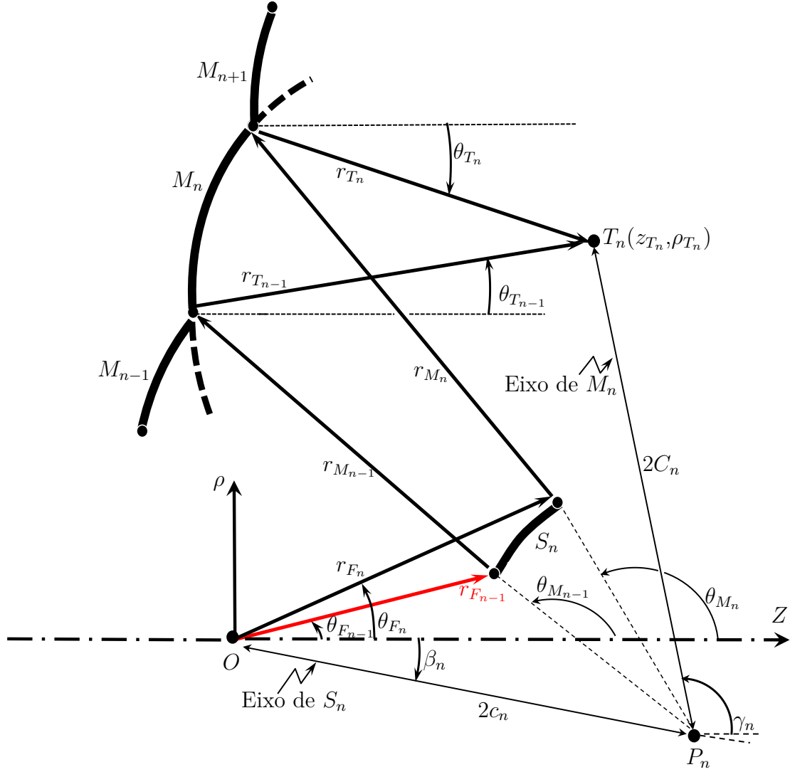
Figura 2.8 – Parametrização geométrica do par de seções cônicas S_n e M_n .
