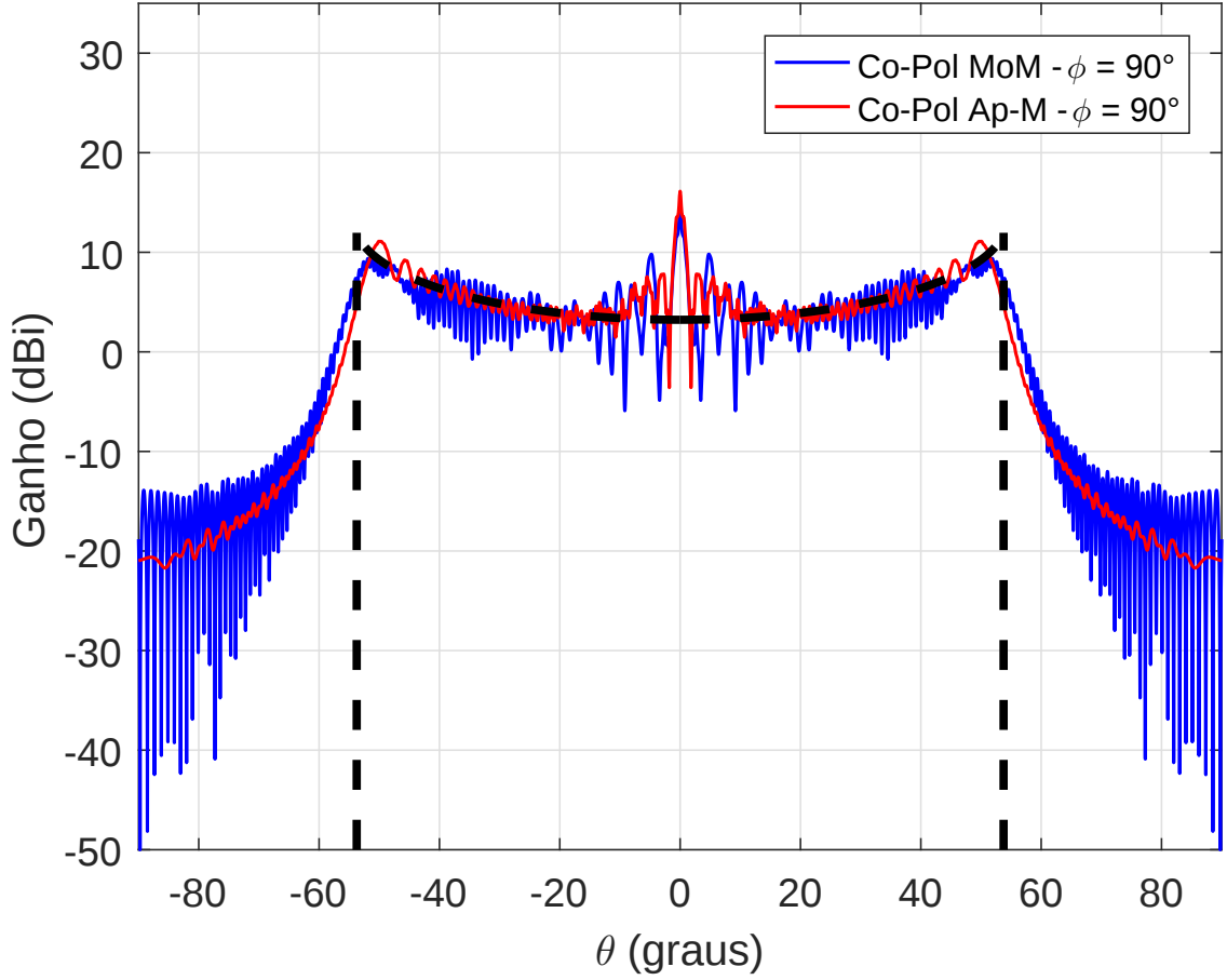
Figura 3.35 – Diagramas de radiação no plano \phi = 90^\circ obtidos via MoM (linha sólida na cor azul) e Ap-M (linha sólida na cor vermelha) para a antena ADC modelada do estudo de caso B.6. Em linhas tracejadas na cor preta está representado o diagrama de radiação isoflux ideal da GO em -53,75^\circ \leq \theta \leq 53,75^\circ .
