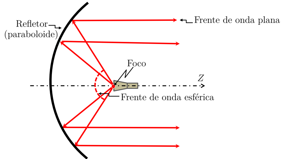
Figura 1.1 – Traçado de raios em uma antena refletora parabólica alimentada pelo foco.
