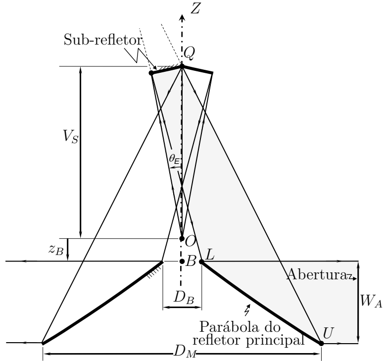
Figura 4.4 – Parametrização geométrica de uma configuração OADH clássica.
