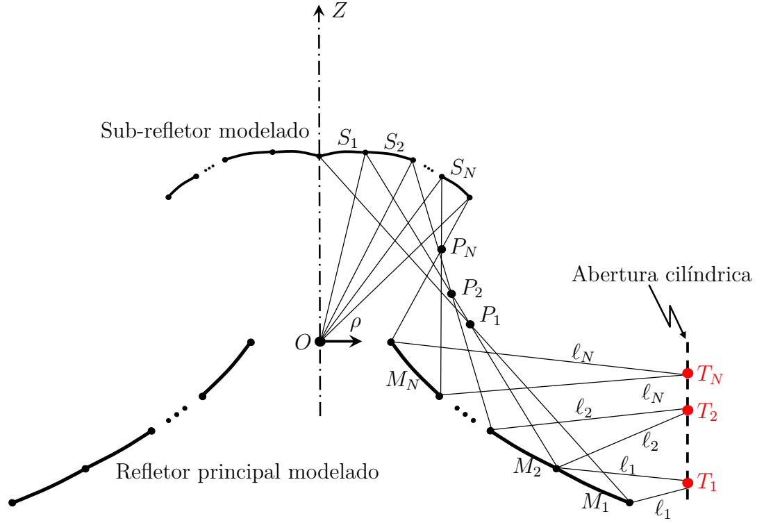
Figura 5.4 – Exemplificação de uma configuração duplo-refletora omnidirecional OADE modelada pela concatenação contínua de seções cônicas com uma abertura cilíndrica, onde \ell_n varia a cada iteração n .
