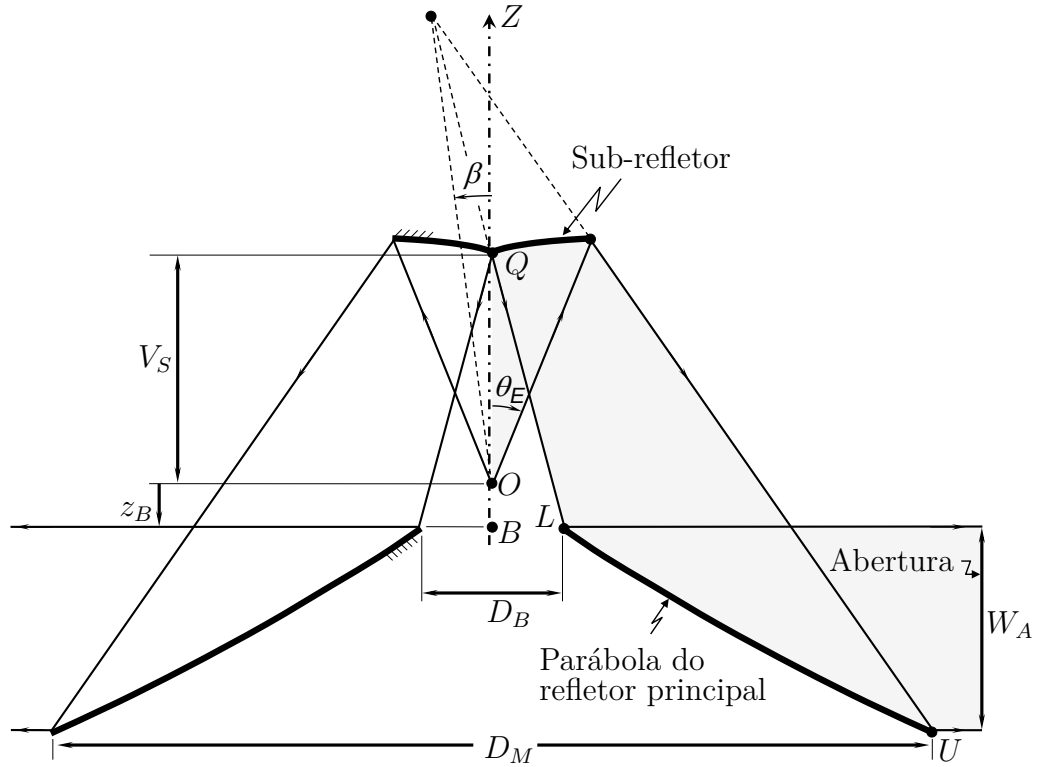
Figura 4.1 – Parametrização geométrica de uma configuração OADC clássica.
