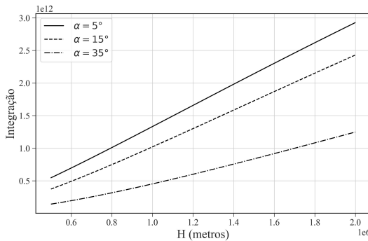
Fig. 5. Comparação entre solução analítica e numérica em função de H para diferentes valores de \alpha_{min} .
