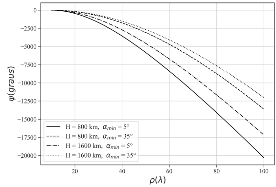
Fig. 6. Comparação entre solução analítica e numérica para distribuição de fase não uniforme para combinações de valores de H e \alpha_{min} .
