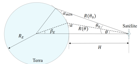
Fig. 3. Posição do satélite em relação à Terra.
